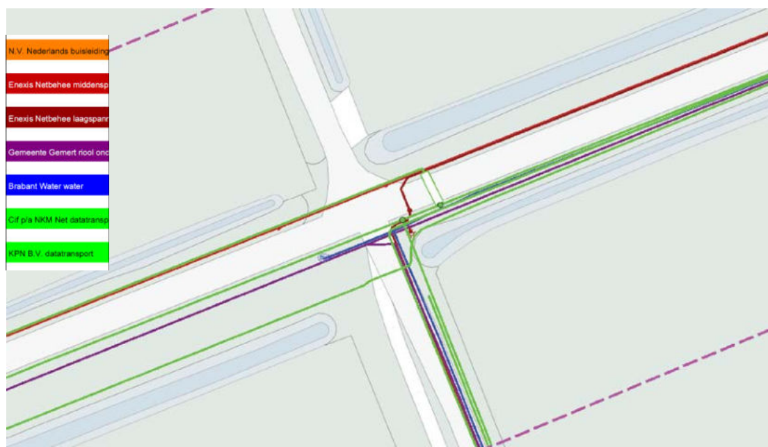
Figuur 4.1: aanwezige kabels en leidingen bij de Nachtegaallaan
