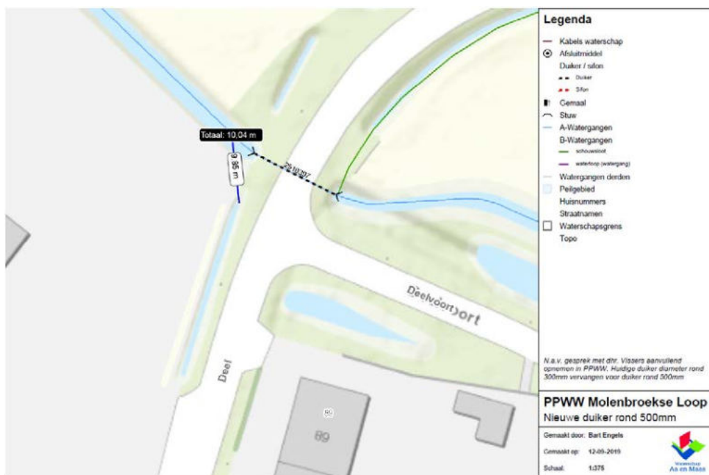
Figuur 2.4 Locatie te vervangen duiker langs Deel
