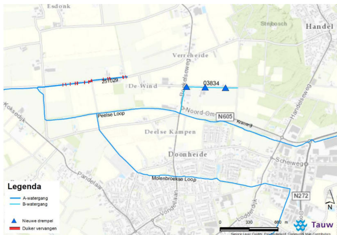
Figuur 2.2 Voorgenomen werkzaamheden
