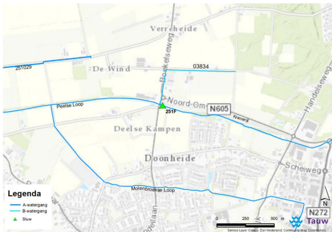
Figuur 2.1 Afwatering watergang 03834
