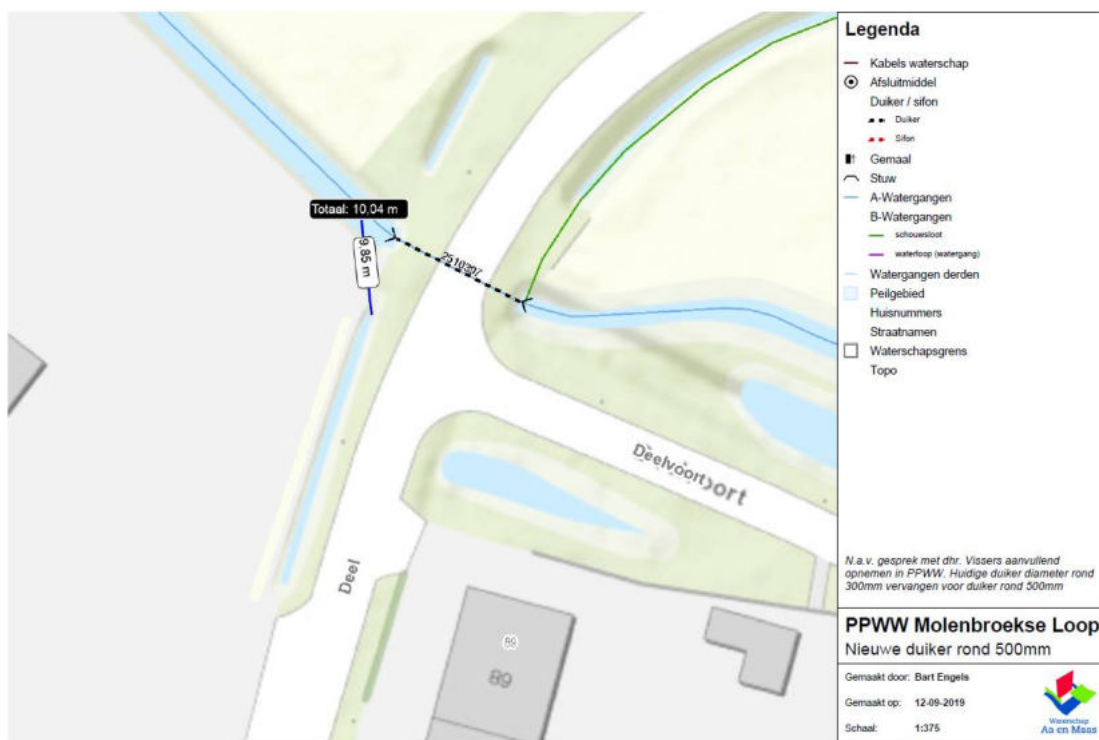
Figuur 4.2: situatietekening nieuwe duiker
