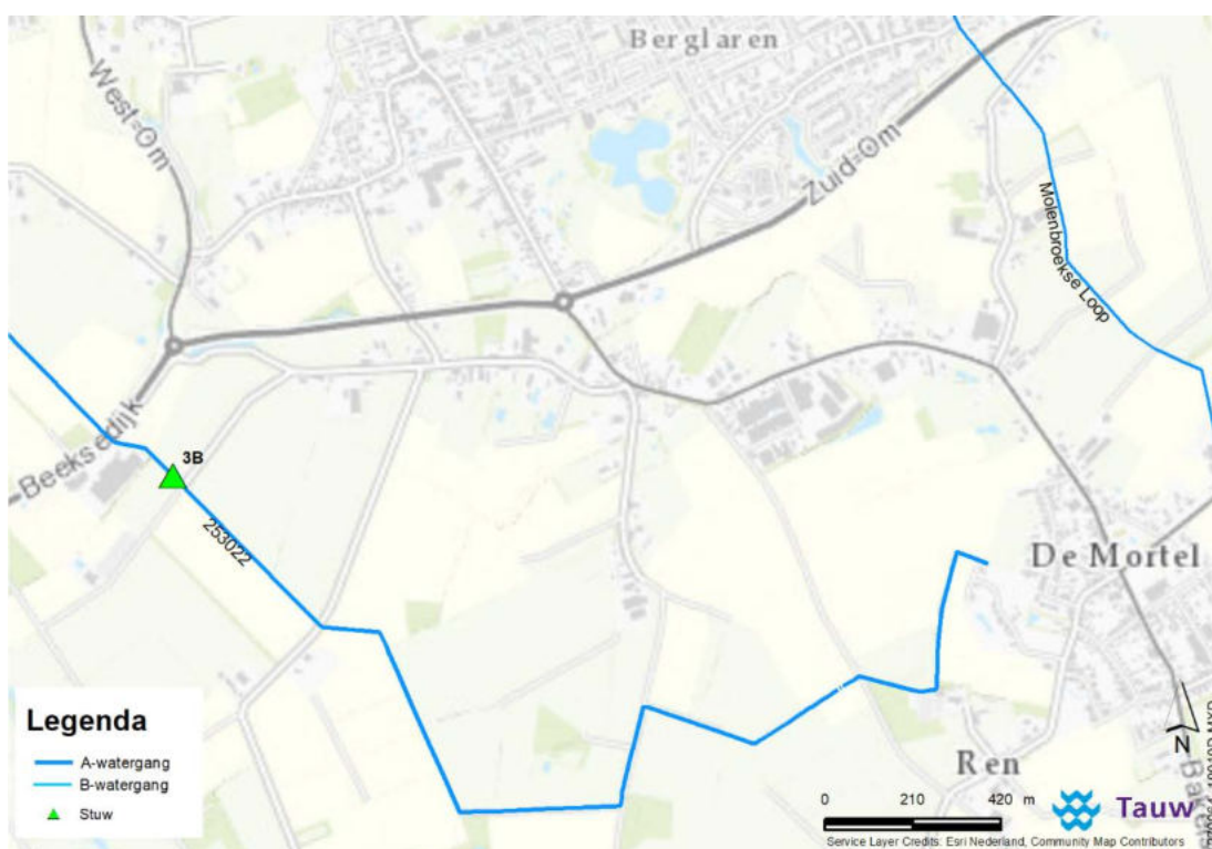
Figuur 3.5 Locatie automatiseren stuw
