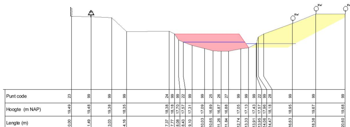
Profiel 251001P1400
