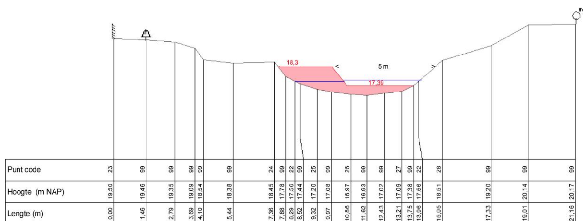
Profiel 251001P1390
