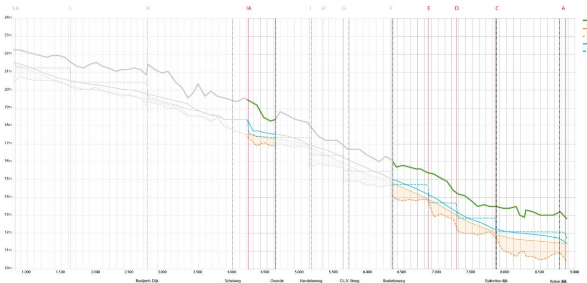
Figuur 5.1a. Huidige en nieuwe zomer waterstanden. Het gedeelte waar dit projectplan betrekking op heeft is gekleurd weergegeven. Oranje lijn = huidige bodem, oranje vlak = bodemophoging, blauwe streepjes lijn = huidige waterstand, blauwe doorgetrokken lijn = nieuwe waterstand, groene lijn = maaiveld direct naast de beek.
