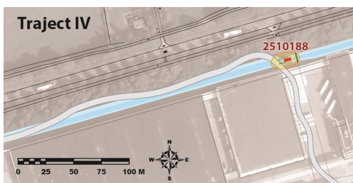
Figuur 3.3.1d1. Ligging duikers in traject IV.
