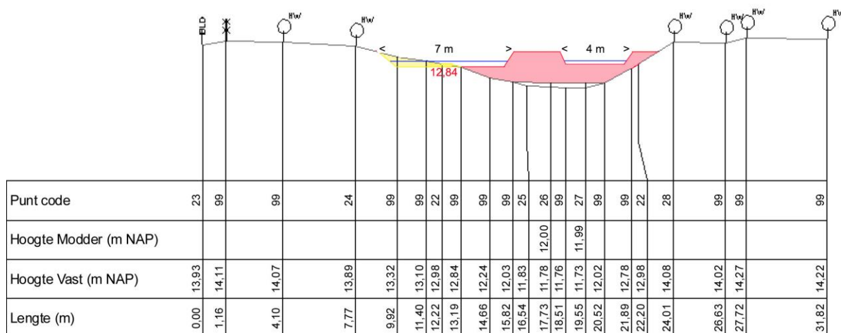
Figuur A.5. Nieuwe doorsnede van de versmalde bedding juist na de instroom van de Molenbroekse loop die hier door de linkerbedding loopt.
