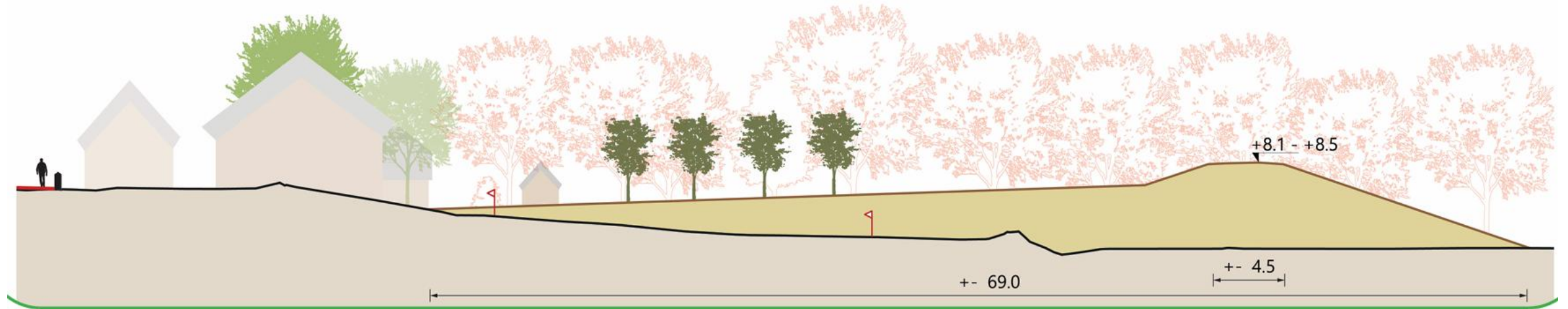
DWARSPROFIEL F OUD-EMPEL
