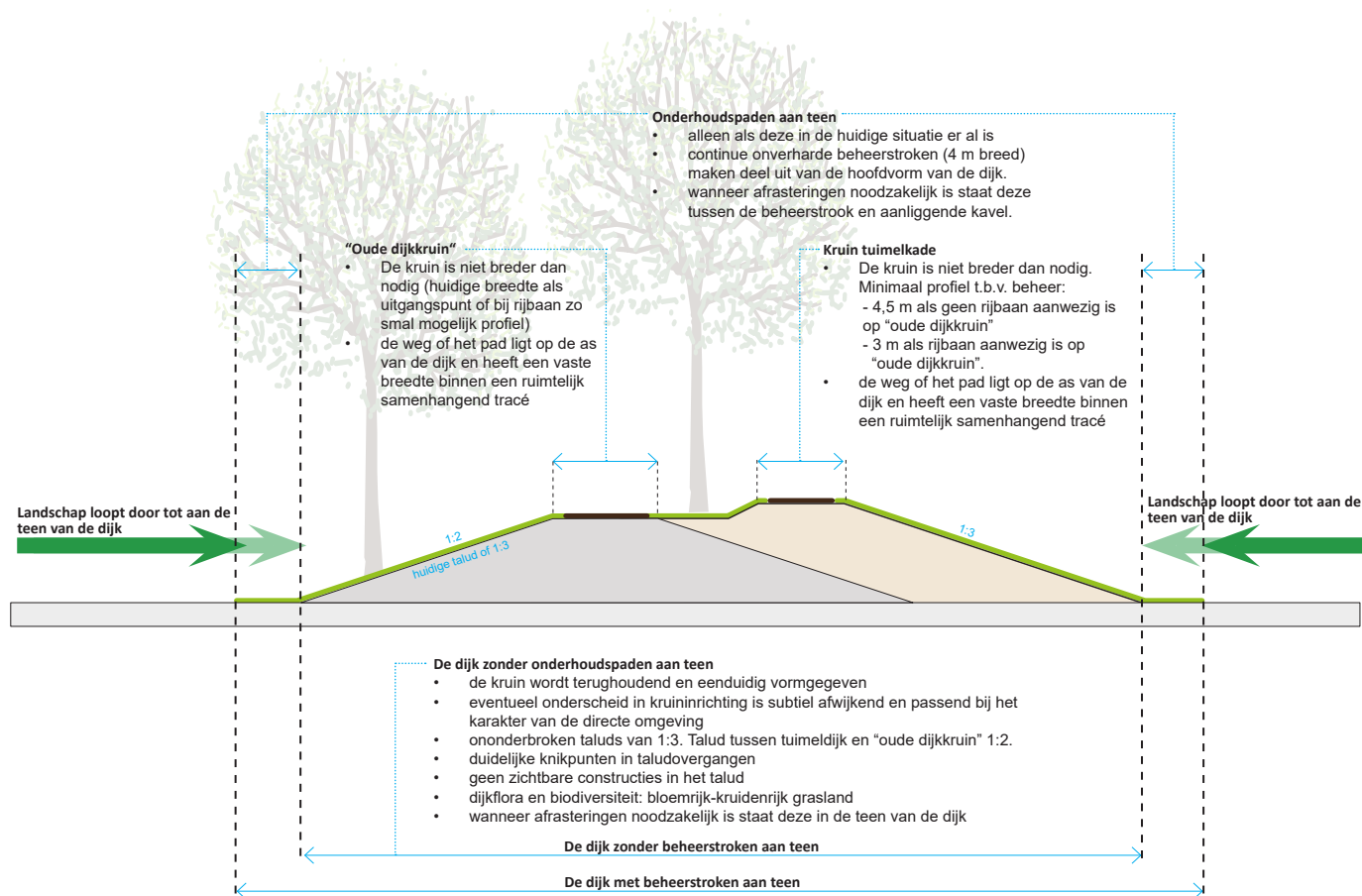
Figuur 28: principeprofiel dijk met tuimelkade.
