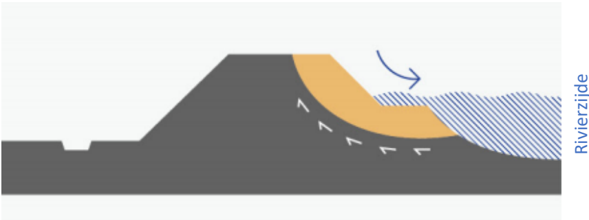
Dijk zakt weg aan rivierzijde (stabiliteit)
