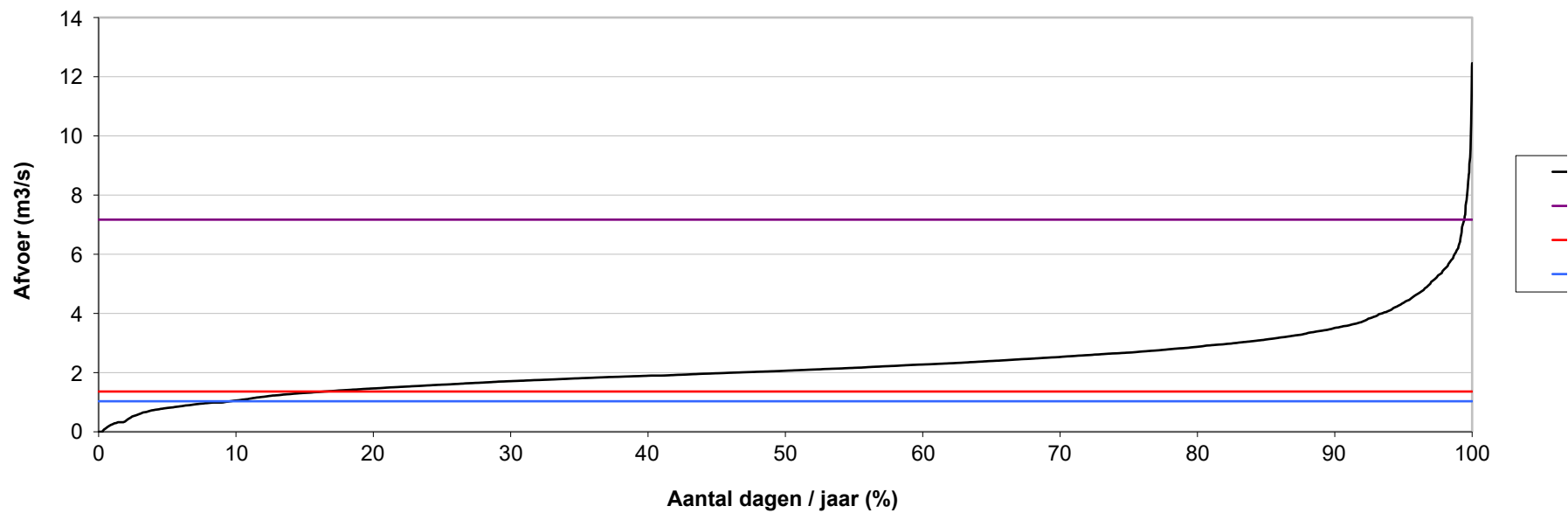
Herhalingstijden afvoeren
