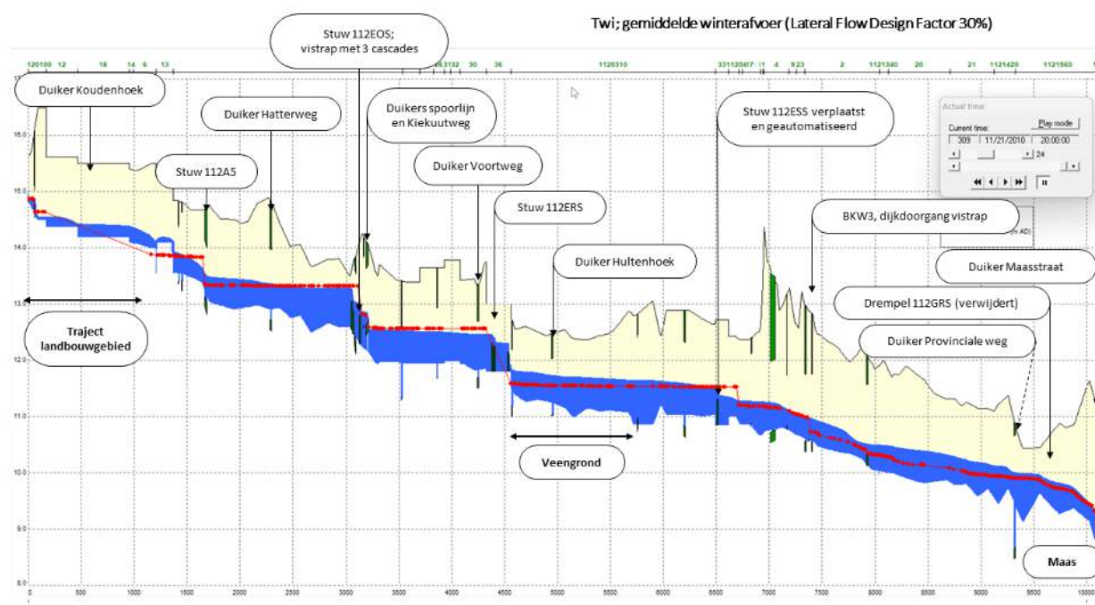
Figuur 22 Langsdoorsnede met waterstand voor een gemiddelde winter afvoer scenario (T100) (blauwe vlak)- en referentiemodel (rode lijn) inclusief bodem- en maaiveldniveau.
