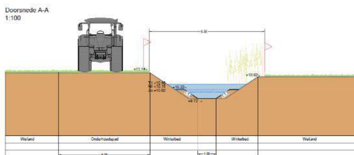
Figuur 10: Basisprofiel 'accoladeprofiel binnen profiel bestaande beek'
