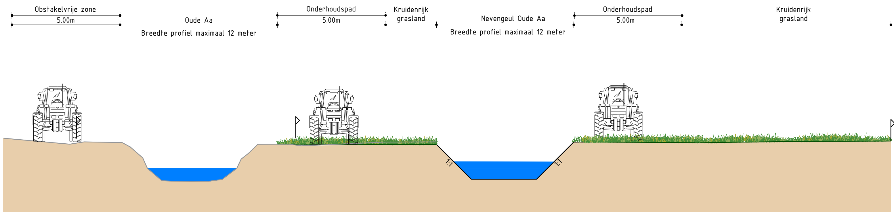
Principeprofiel Oude Aa1 (OA1) (NVO+EVZ)
