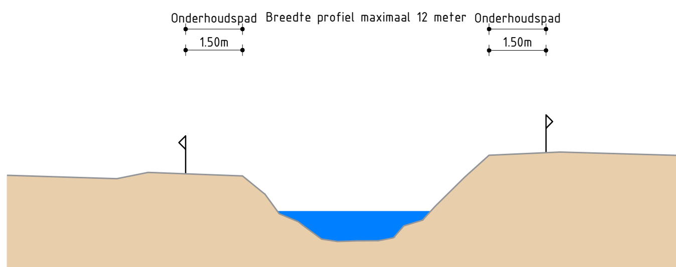
Principeprofiel bestaande situatie
