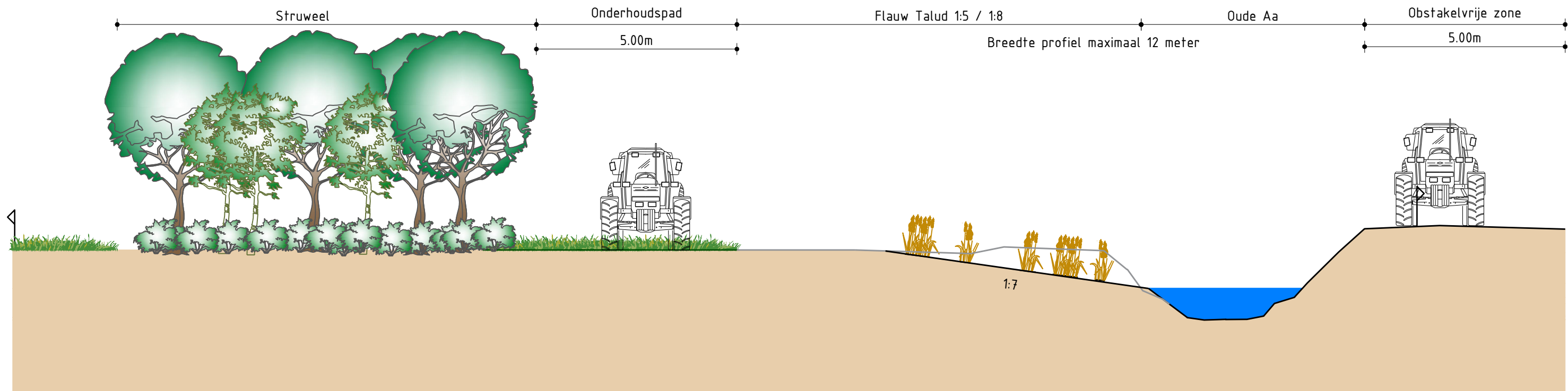
Principeprofiel Oude Aa (NVO+EVZ)
