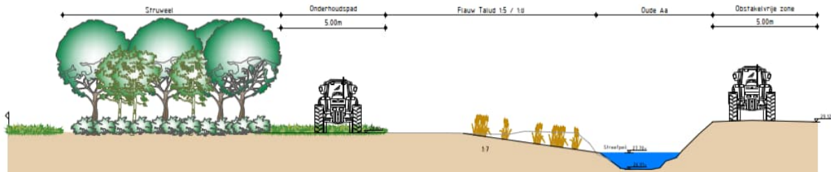
Figuur 7: Principeprofiel Oude Aa (NVO + EVZ)
