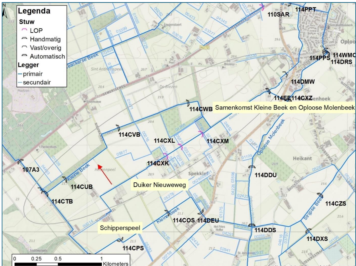
Figuur 1-1 Watersysteem cluster 1, deelgebied Kleine Beek-Spekkleef (rode pijl geeft afvoerrichting van het deelstroomgebied Schipperspeel in de praktijk weer)
